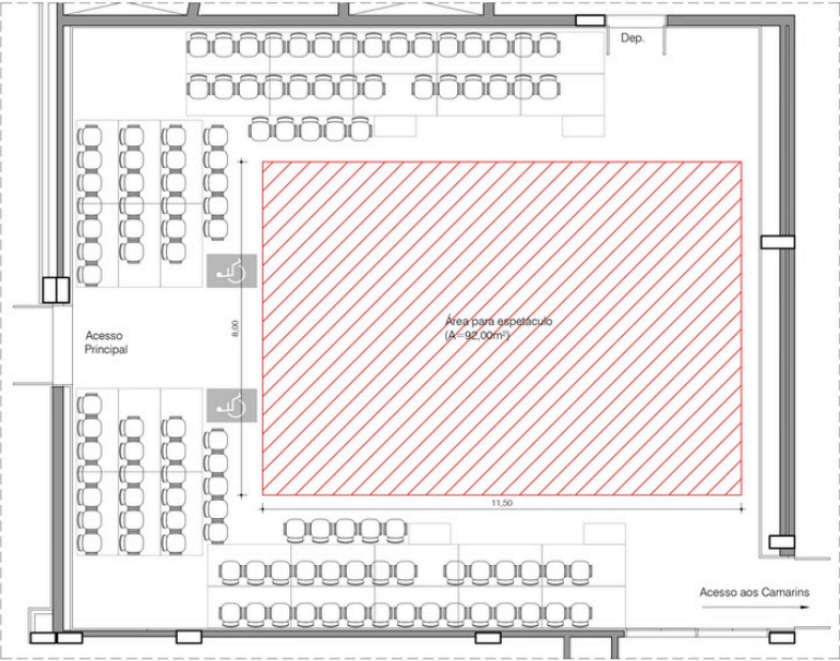
PLANTA BAIXA - PALCO E PLATEIA 116 CADEIRAS + 2 PCDs = 118 LUGARES
